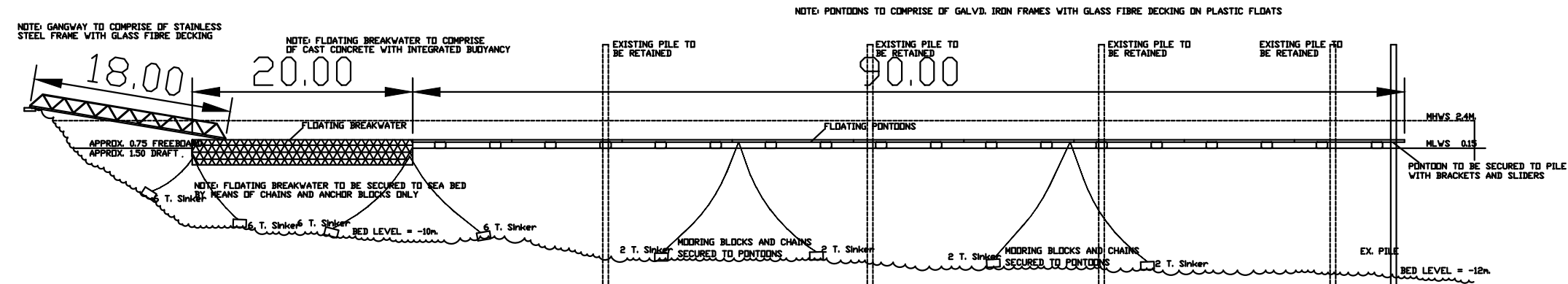
SECTION A-A
