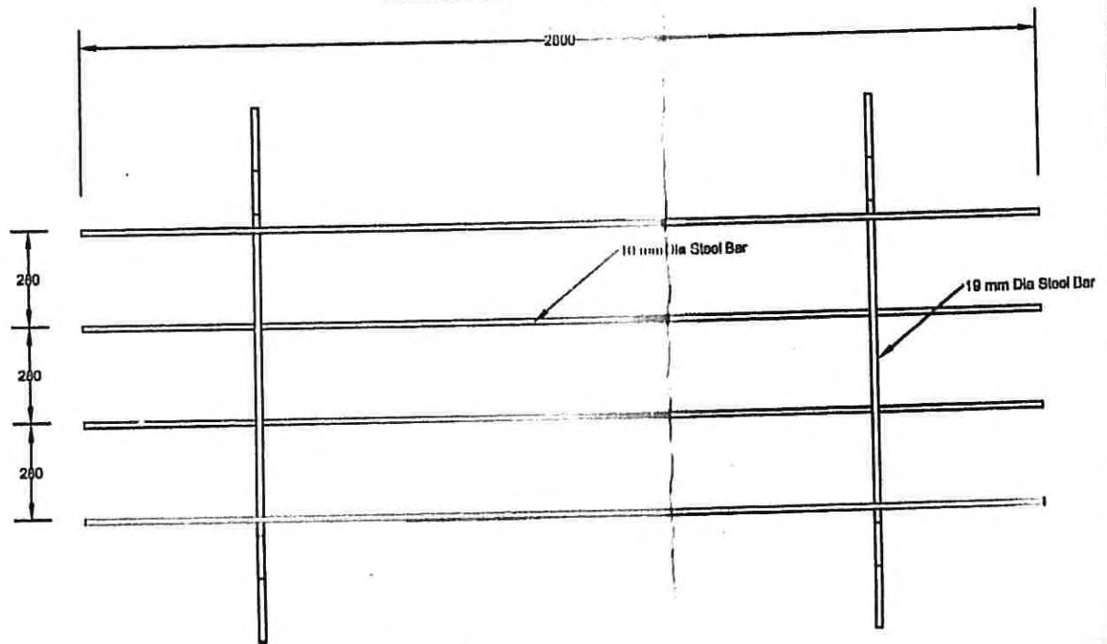
LONGITUDINAL SECTION
