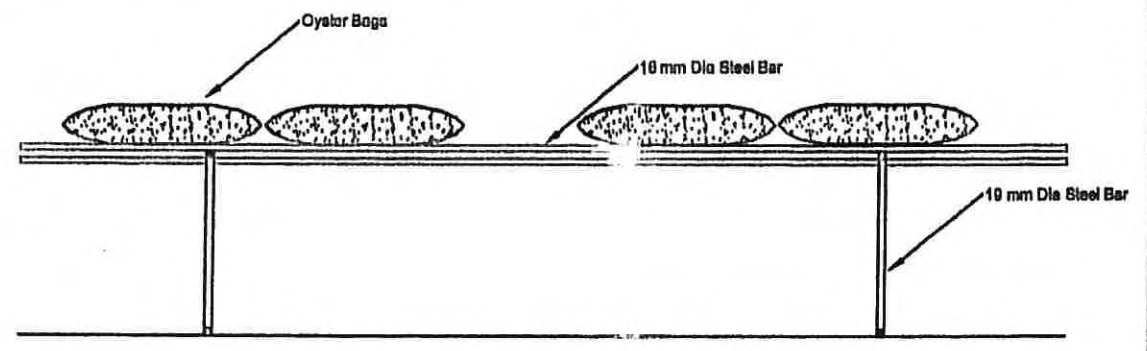
LONGITUDINAL SECTION
